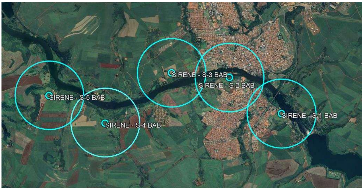
Figura 34 – Localização das Estações Remotas (ER) de Sirenes Fixas na ZAS
