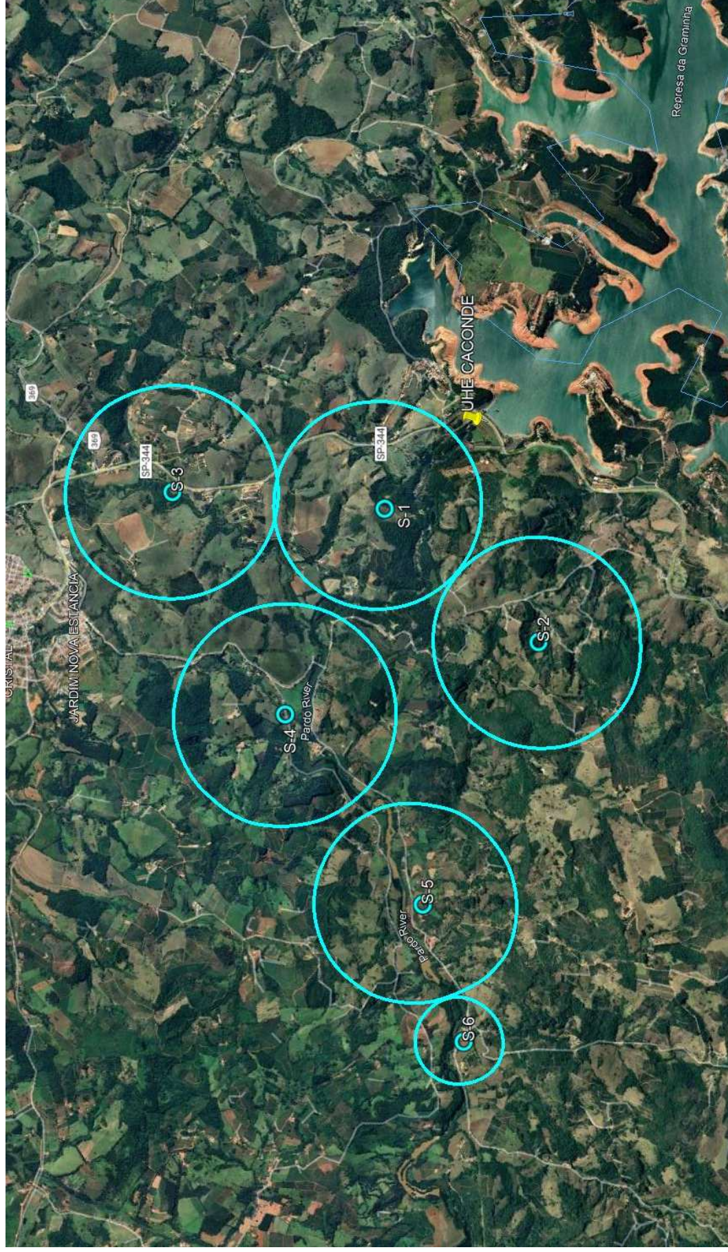
Figura 27 – Localização das Estações Remotas (ER) de Sirenes Fixas na ZAS
